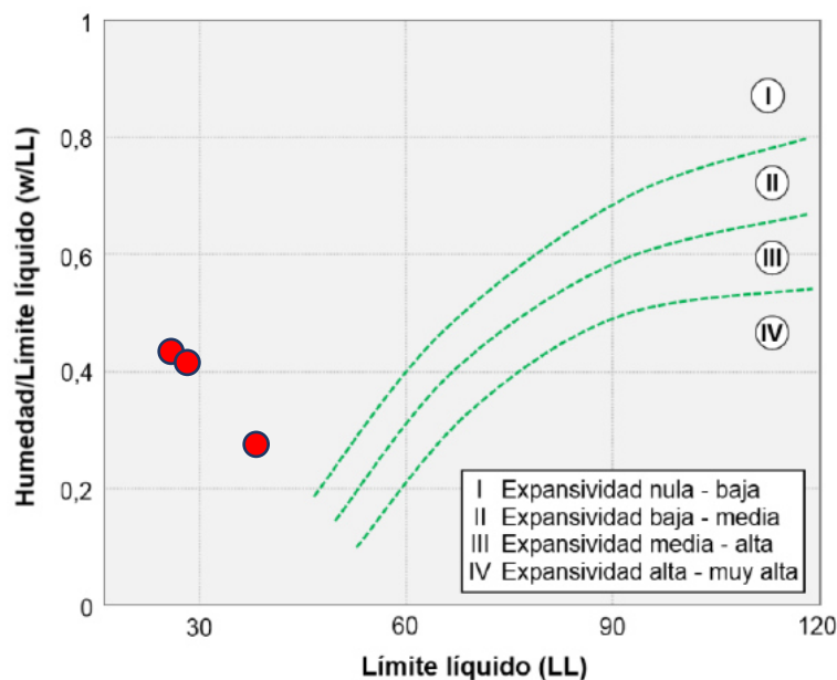
Figura 5: Criterio de peligrosidad a partir de la expansividad (Oteo, 1986).
