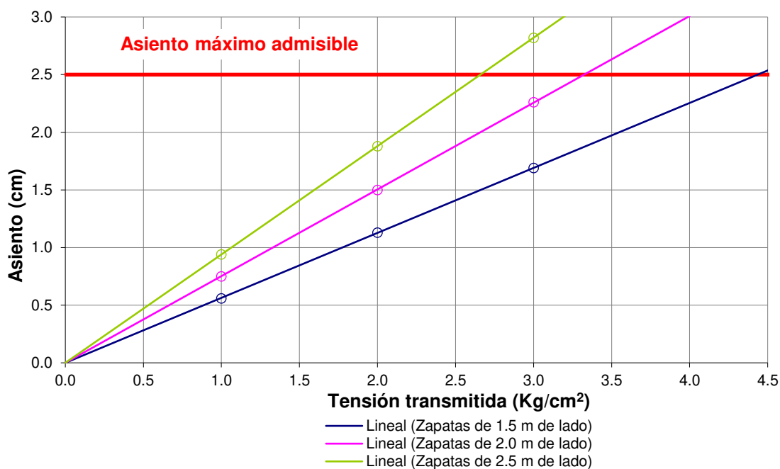
Gráfico 1: Zapatas aisladas apoyadas sobre el Nivel I. Tensión admisible V.S. Asiento
