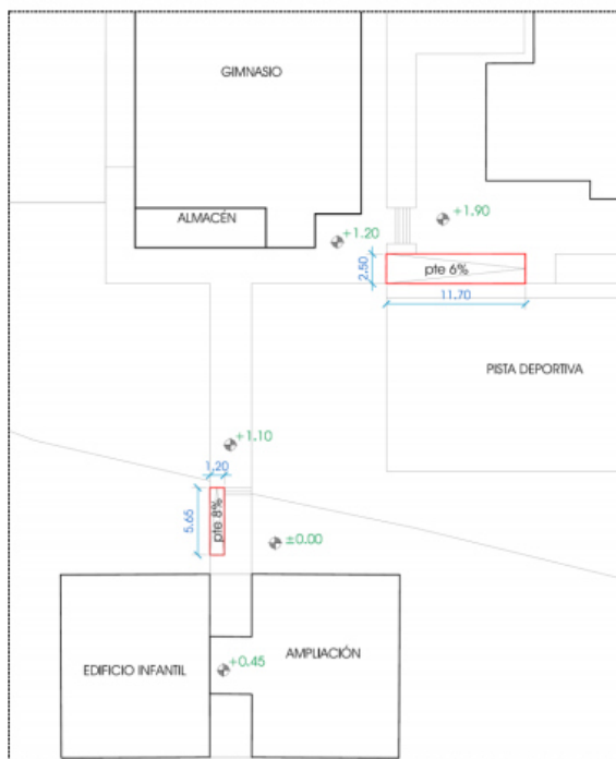
Figura 1: Plano de implantación del nuevo edificio de gimnasio-almacén y la ampliación de las aulas de infantil.
