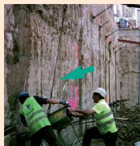
Utilización de medio mecánico para la colocación del gato.
